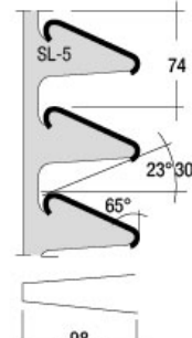
ESTRUCTURA SL5
