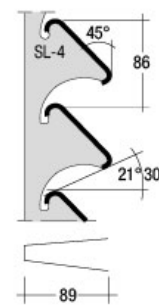
ESTRUCTURA SL4
