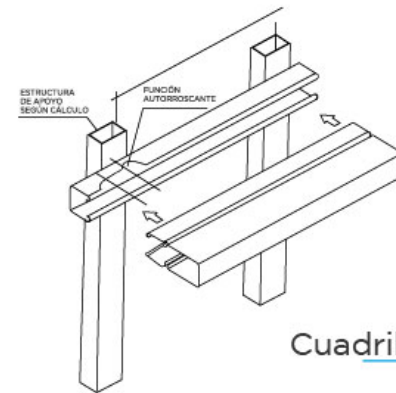
ESTRUCTURA SL4
